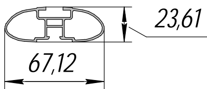
АП-87 АПС; 0,744 кг/п.м.
