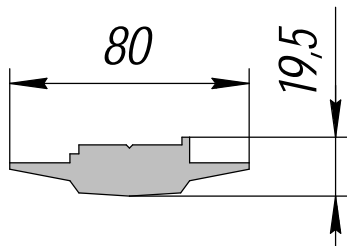
HP-361; 2,172кг/п.м.
