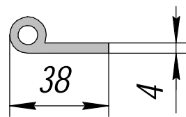
АП-95 ПКФ; 1,136 кг/п.м.
