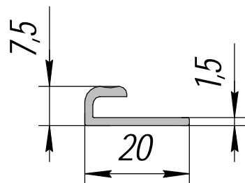
НП-631; 0,134кг/п.м.
