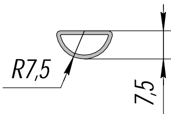
АП-75 ВМ-А; 0,093 кг/п.м.
