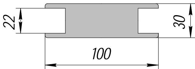
HP-437; 5,975кг/п.м.
