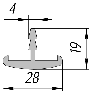
ПК 02090-1; 0,383кг/п.м.
