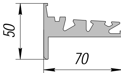
НП-266; 2,624кг2/п.м.
