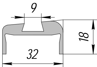
ПК 02090-5; 0,499кг/п.м.
