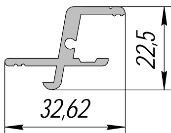
ПА-57; 0,376кг/п.м.
