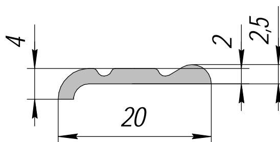
HP-435; 0,104кг/п.м.
