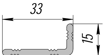
HP-406; 0,328кг/п.м.
