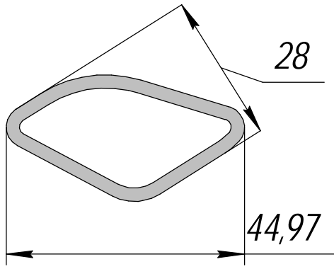
HP-540; 0,669кг/п.м.
