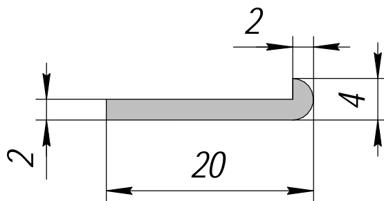
HP-424; 0,115кг/п.м.
