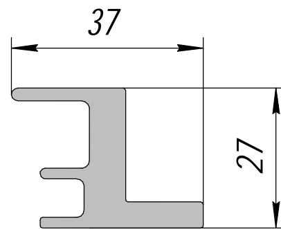
HP-507; 0,942кг/п.м.
