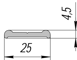
HP-426; 0,424кг/п.м.
