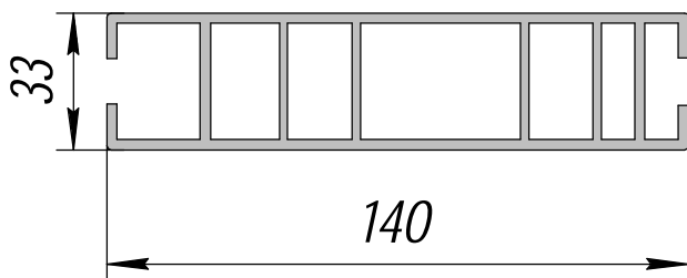
ПК 02090-6; 3,108кг/п.м.
