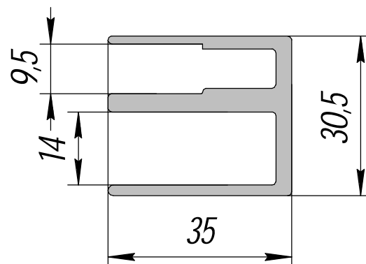
ПК 02170; 0,929кг/п.м.
