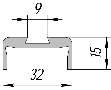
ПК 02090-4; 0,430кг/п.м.
