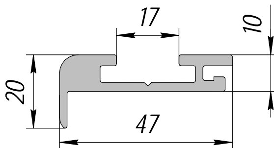
HP-509; 0,757кг/п.м.
