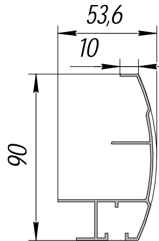
АП-72; 0,788 кг/п.м.
