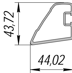
АП-39-01 АПС; 0,871кг/п.м.
