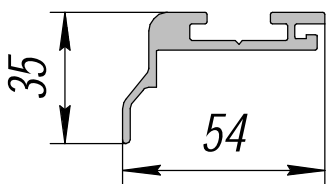
АП-90 Нефаз; 0,869 кг/п.м.
