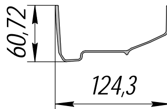
ПА-62-01; 1,361кг/п.м.
