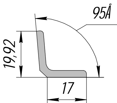
ПВ 1717; 0,292кг/п.м.
