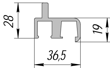
HP-387; 0,869кг/п.м.
