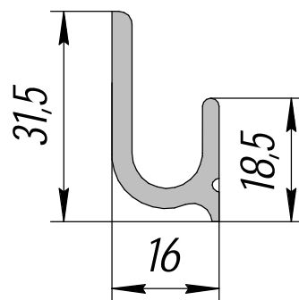
HP-426; 0,424кг/п.м.
