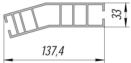
AC-79; 3,047кг/п.м.
