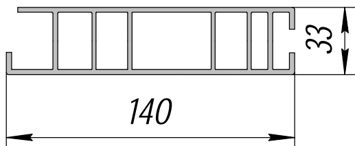
AC-80; 3,015кг2/п.м.
