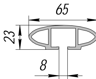
АП-45; 1,156 кг/п.м.
