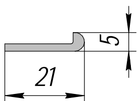
АПР 291-2; 0,153кг/п.м.
