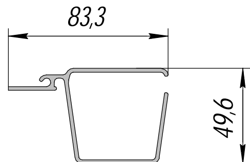
АП-74 ВМ-А; 1,176 кг/п.м.
