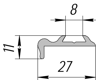
HP-518; 0,708кг/п.м.
