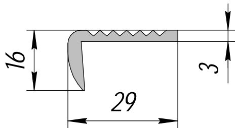
НП-603; 0,292кг/п.м.
