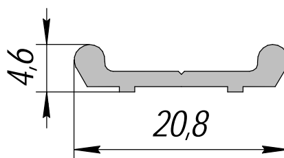
ПА-61; 0,118кг/п.м.
