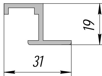
ПК 02082; 0,319кг/п.м.
