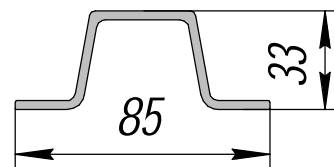
АП-41 АПС; 1,083кг/п.м.
