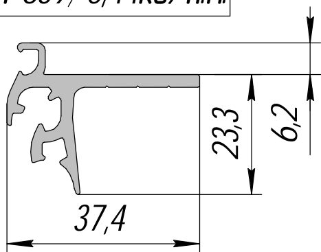
НП-640; 0,52кг/п.м.
