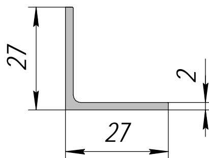
НП-637; 0,284кг2/п.м.
