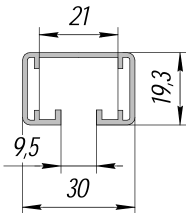
АП-70; 2,323 кг/п.м.
