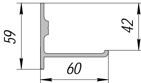
КП-2042; 1,115кг2/п.м.
