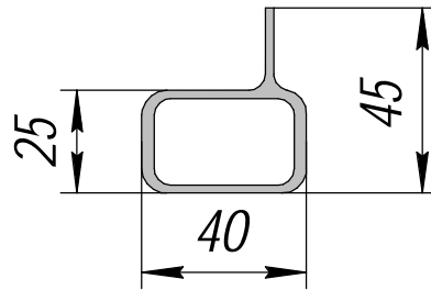
ПК 02090-8; 0,858кг/п.м.
