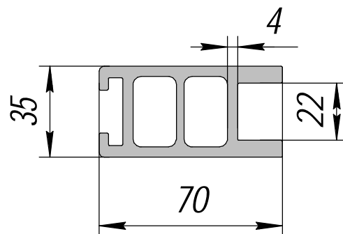
ПА-090; 0,312кг/п.м.
