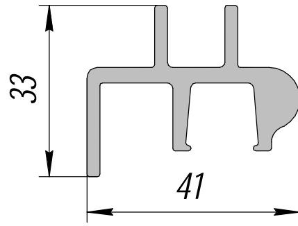
HP-590; 0,926кг/п.м.
