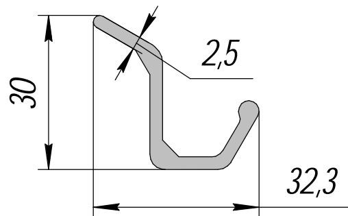
ПК 02105; 0,442кг/п.м.
