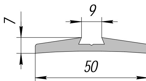
ПК 02090-2; 0,606кг/п.м.
