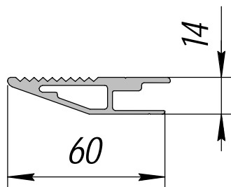
АП-48 АПС; 0,901 кг/п.м.
