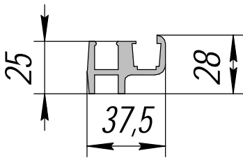
HP-360; 0,901кг/п.м.
