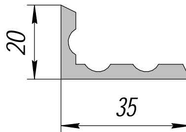
HP-377; 0,451кг/п.м.
