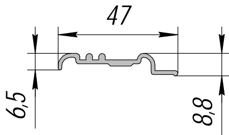
HP-324; 0,295кг/п.м.
