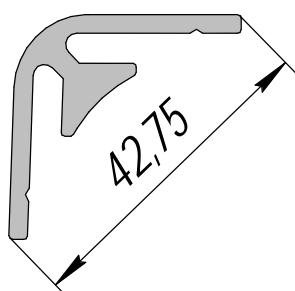
ПА-54; 0,539кг/п.м.
