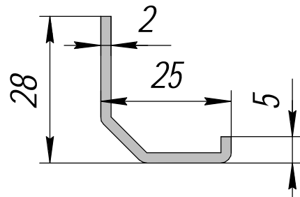
HP-595; 0,266кг/п.м.
