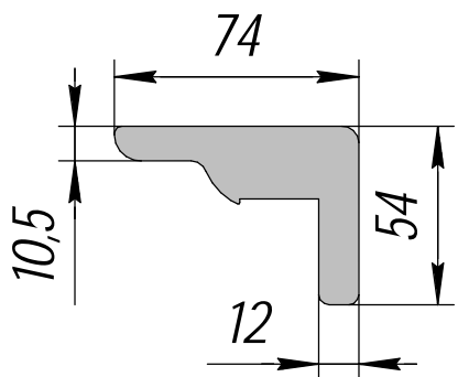
АП-76 АПС; 4,482 кг/п.м.
