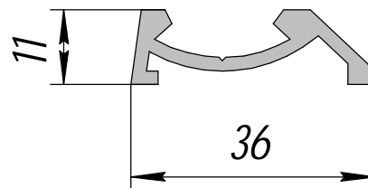
HP-366; 0,356кг/п.м.
