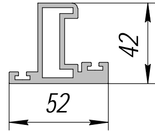
AC-76; 1,460кг/п.м.
