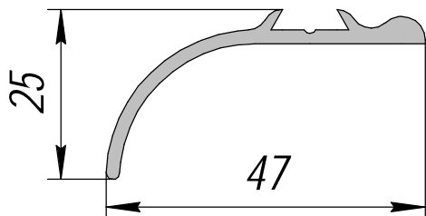
HP-408; 0,366кг/п.м.
