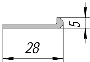
АПР 291-1; 0,169кг/п.м.
