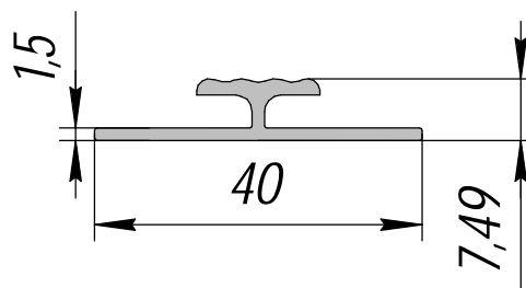
ПА-63; 0,256кг/п.м.
