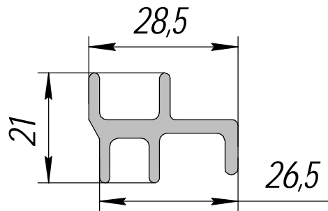
HP-401; 0,466кг/п.м.
