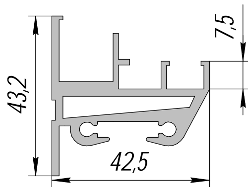
HP-509; 0,757кг/п.м.
