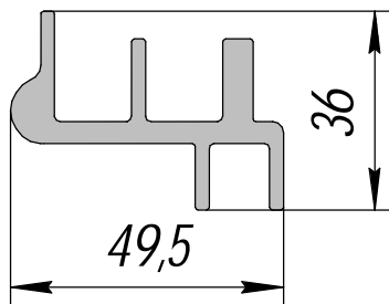
HP-588; 1,24кг/п.м.
