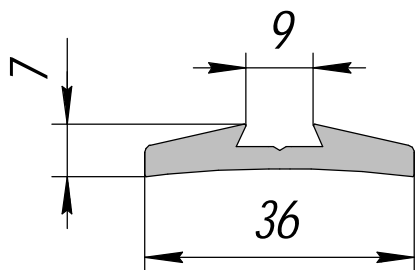
АПР 323; 0,131кг/п.м.
