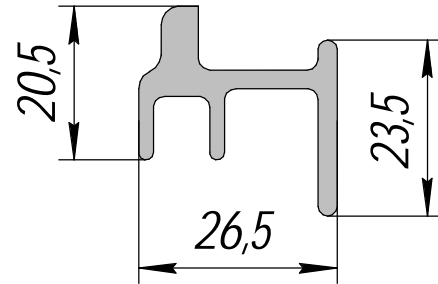
HP-400; 0,557кг/п.м.
