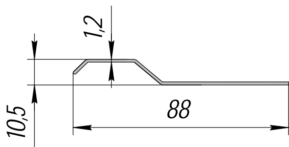
HP-505; 0,303кг/п.м.
