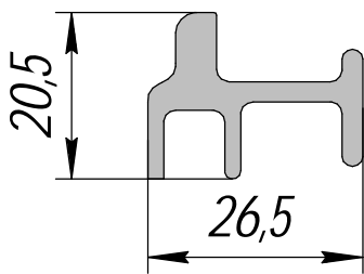
HP-404; 0,498кг/п.м.
