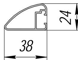
АП-88; 0,433 кг/п.м.
