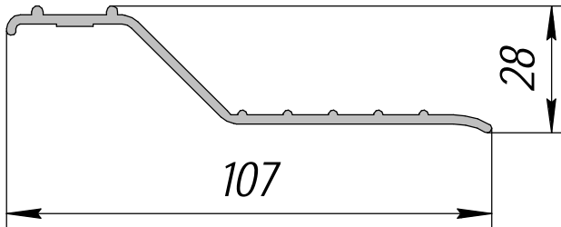
HP-325; 0,692кг/п.м.
