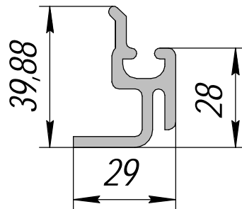
HP-385; 0,828кг/п.м.
