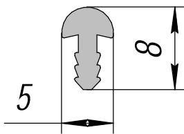
AC-69; 0,059кг/п.м.
