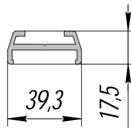
АП-82 Лицз; 0,557 кг/п.м.
