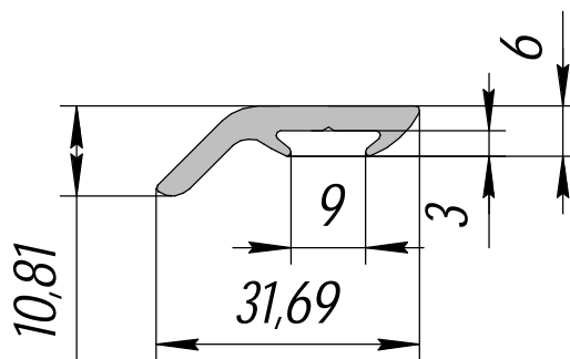
HP-425; 0,311кг/п.м.
