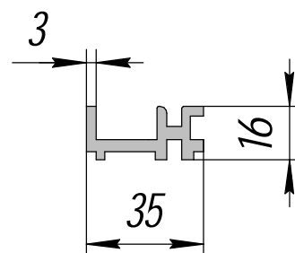
HP-367; 0,663кг/п.м.
