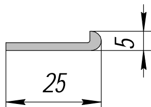
АПР 291-2; 0,153кг/п.м.
