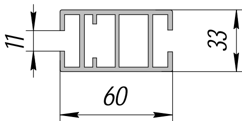
ПК 02090-7; 1,623кг/п.м.
