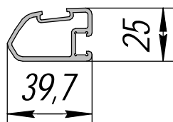
АП-77 АПС; 0,673 кг/п.м.
