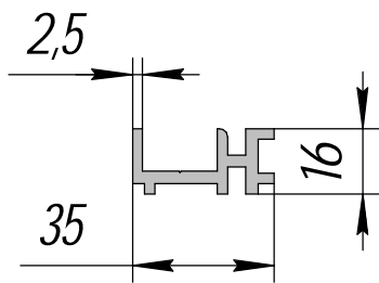
HP-367-01; 0,586кг/п.м.
