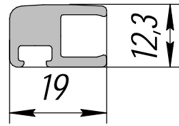
HP-397; 0,352кг/п.м.
