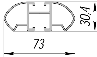
АП-95 ПКФ; 1,136 кг/п.м.
