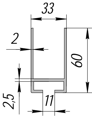
AC-65; 3,149кг/п.м.
