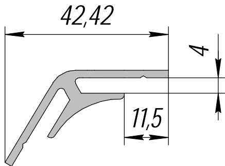
HP-587; 0,491кг/п.м.
