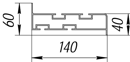
АП-81; 2,521 кг/п.м.
