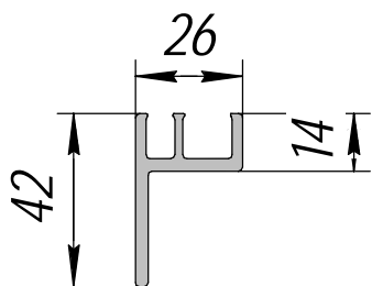
АП-78; 0,652 кг/п.м.
