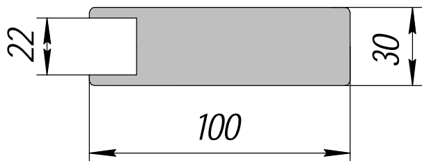
HP-438; 7,047кг/п.м.
