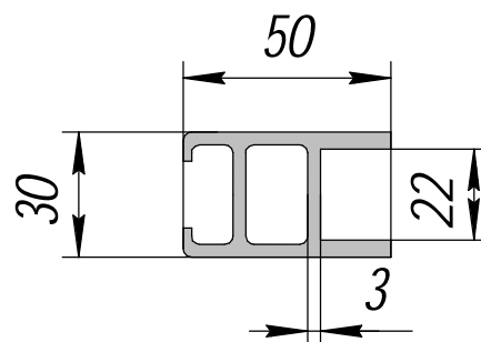
HP-435; 0,104кг/п.м.
