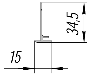
HP-374; 0,22кг/п.м.
