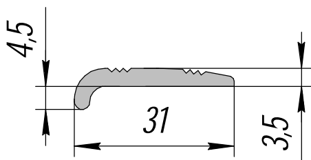
HP-405; 0,279кг/п.м.
