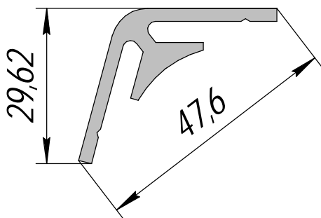
ПА-53; 0,595кг/п.м.
