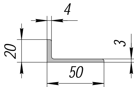
ПК 111-17; 0,591кг/п.м.
