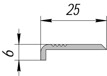
HP-369; 0,140кг/п.м.
