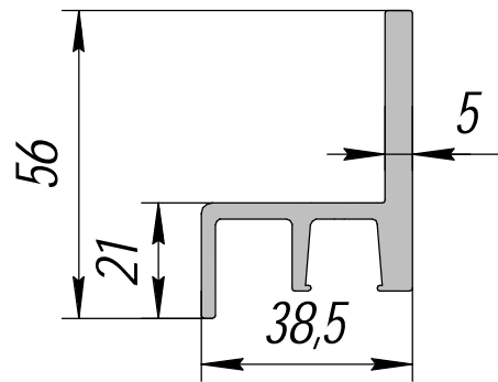
HP-593; 1,227кг/п.м.
