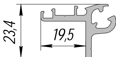
НП-639; 0,44кг/п.м.
