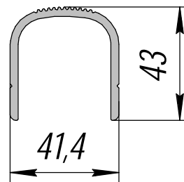
АП-97 Нефаз; 0,879 кг/п.м.
