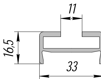
ПК 02090-3; 0,433кг/п.м.
