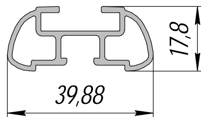
АП-100; 0,879 кг/п.м.
