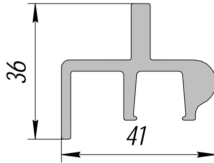
HP-591; 0,966кг/п.м.
