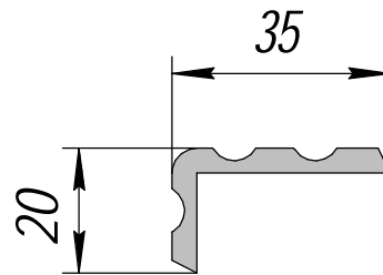
HP-374; 0,22кг/п.м.
