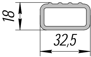
HP-570; 0,595кг/п.м.
