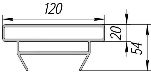
AC-65; 3,149кг/п.м.
